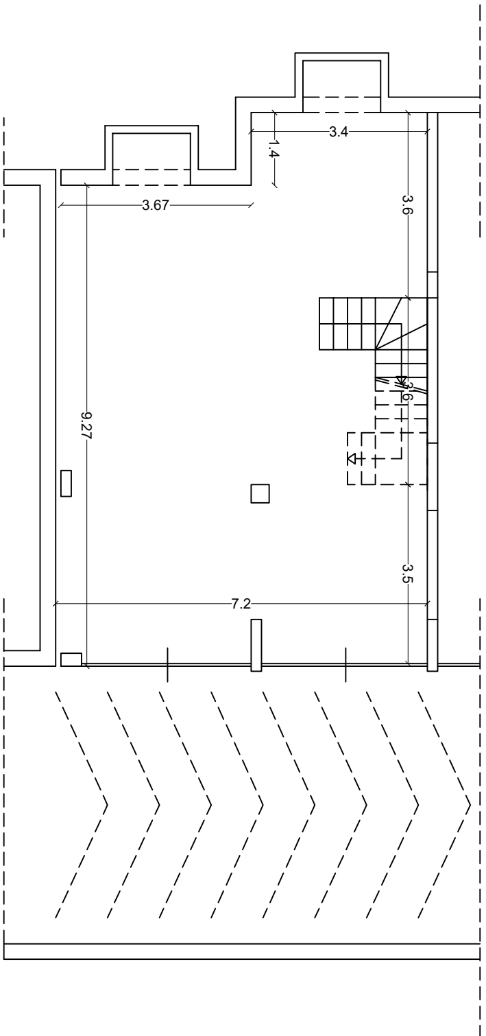
PIANTA PIANO INTERRATO
